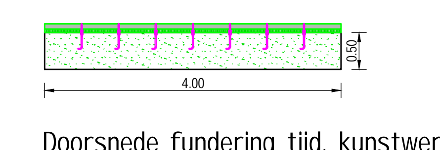
Doorsnede fundering tijd. kunstwerk
