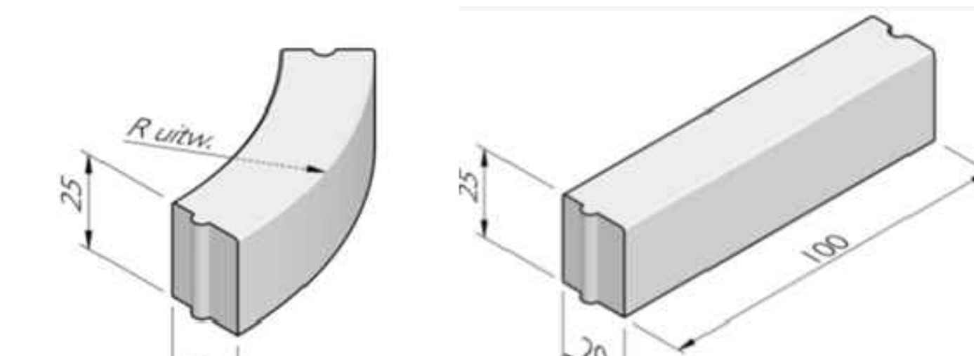
Struyk Verwo opsluitbanden rijloper
